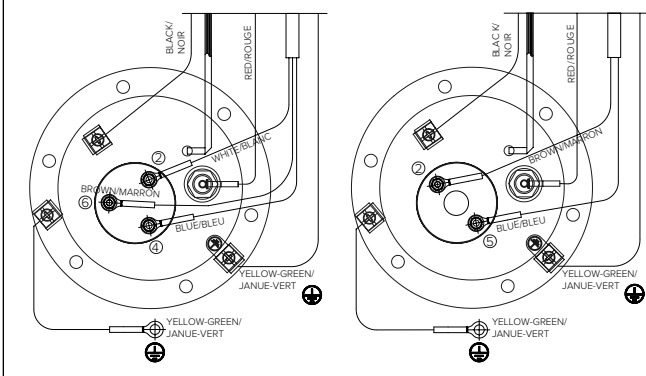
* Possibili configurazioni della resistenza
