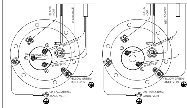
* Possíveis configurações da resistência
